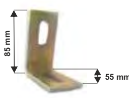
UCHWYT REGULOWANY 30x6 mm, M8 OCYNK na 1 rolkę prowadzącą
