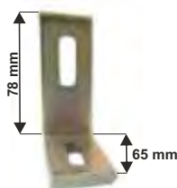
UCHWYT REGULOWANY 40x6 mm, M10 OCYNK na 1 rolkę prowadzącą
